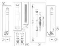
Repuestos horquilla delantera homologado
